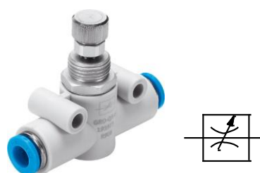
Illustration limiteur de débit FESTO type GRO-QS-4
