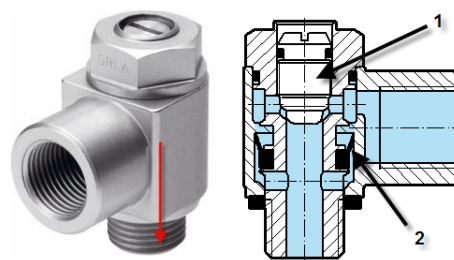
Fig. 23. Régulateur de vitesse FESTO type GRLZ-1/8-B
