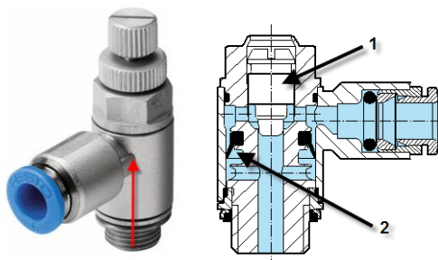
Fig. 22. Régulateur de vitesse FESTO type GRLA-1/8-QS-4-RS-D
