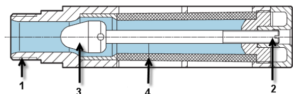
Fig.19. Illustration limiteur de débit FESTO type GRU-1/8-B
