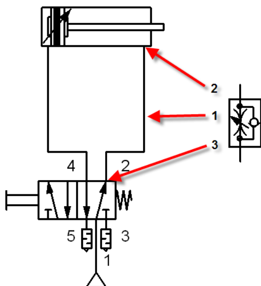
Fig. 20 1: Montage entre distributeur et vérin 2: Montage sur le vérin 3: Montage sur le distributeur
